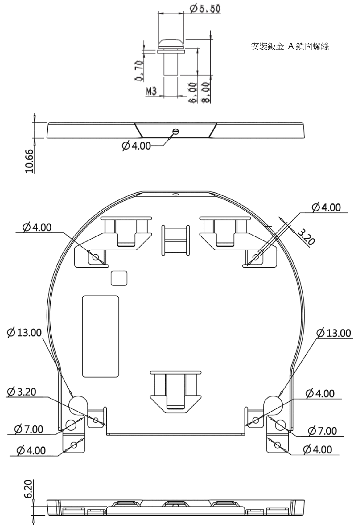
安裝鈹金 A-主機側
